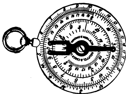
FIG. 15.—CHARPENTIER CALCULIMETRE.
